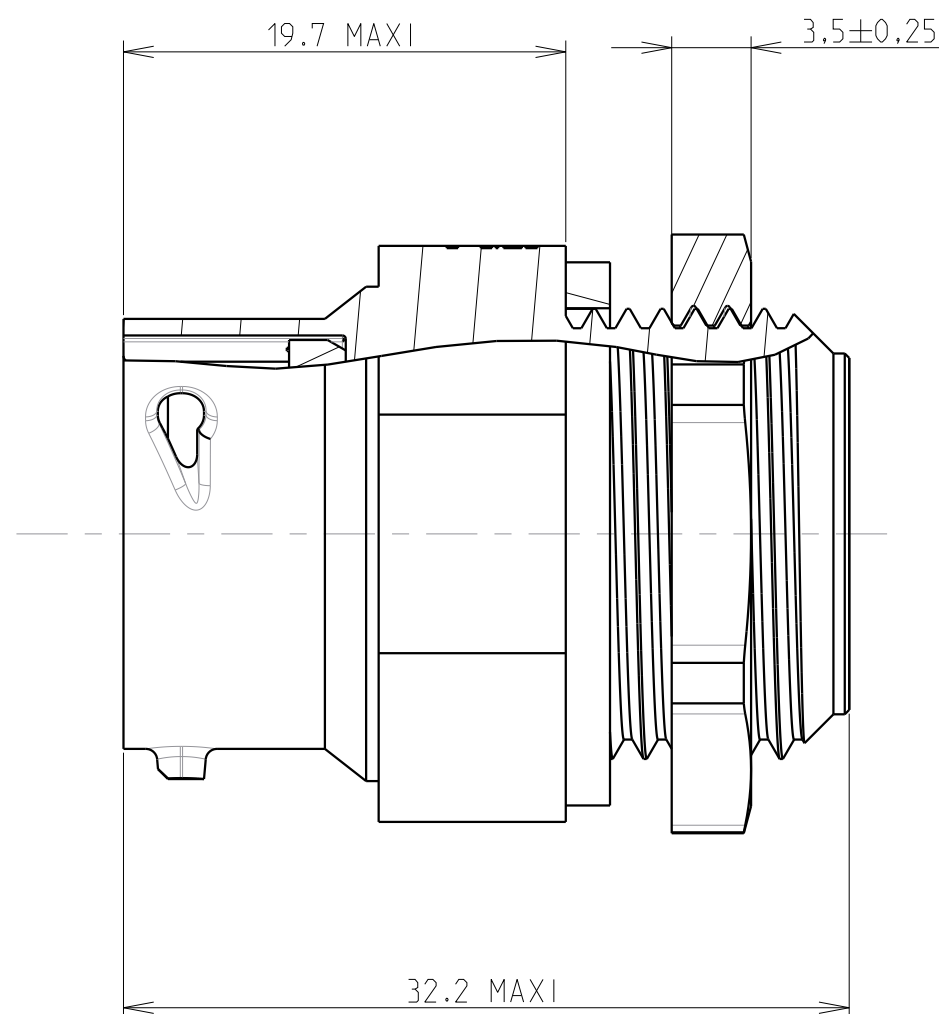
COUPE A-A
